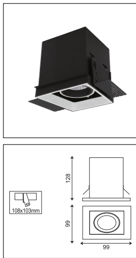
A - Ø 108X99*128mm
